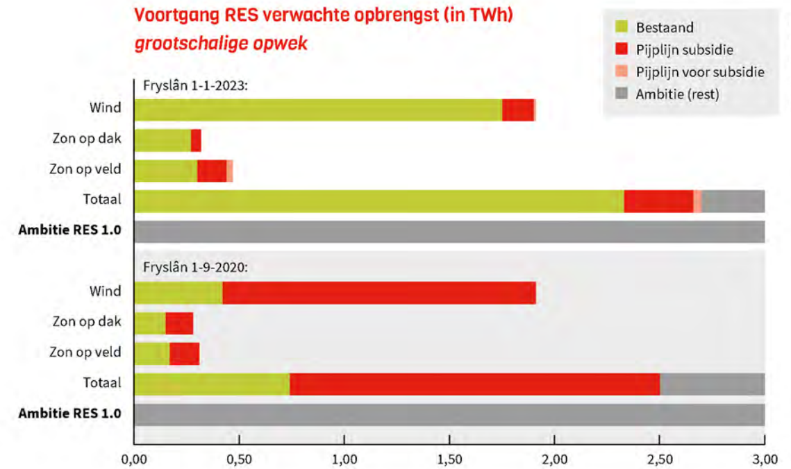
Figuur 1 Voortgang RES Verwachte opbrengst (in TWh) grootschalige opwek
